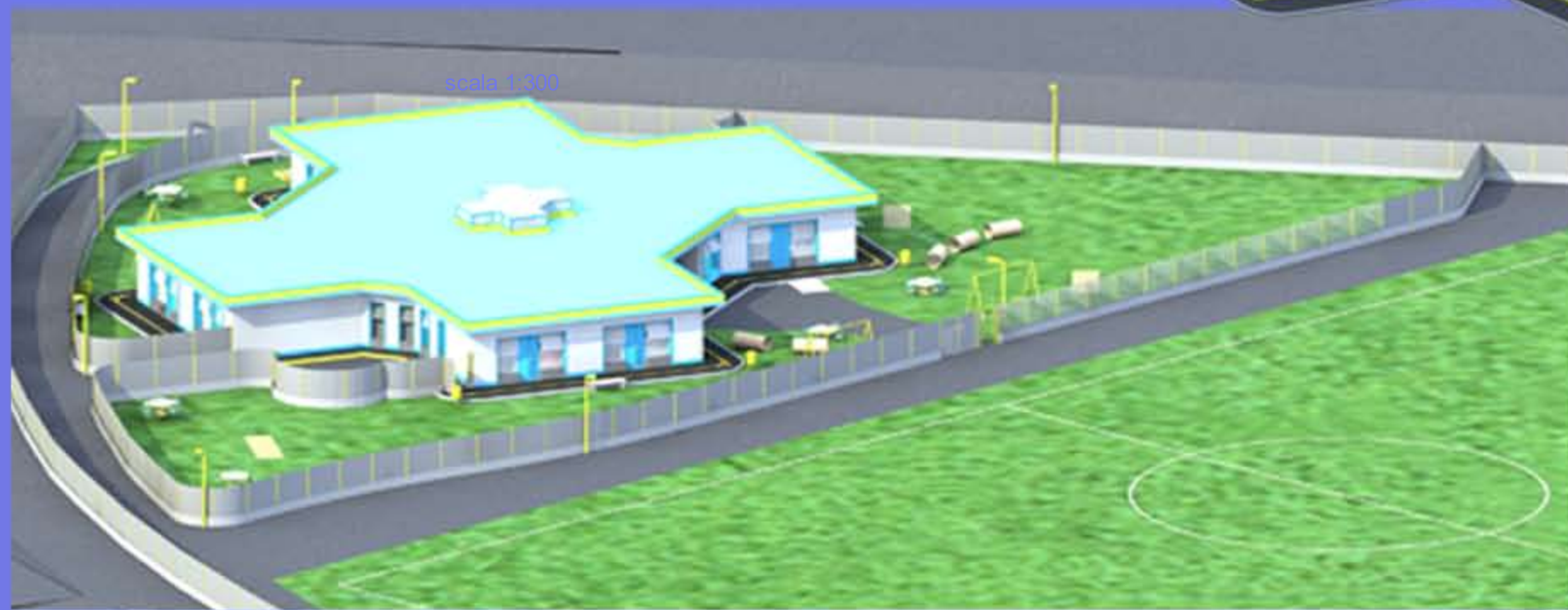
Prospetto Nord-Ovest
